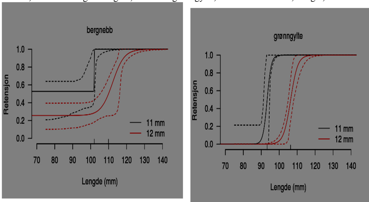
Figur 6. 11 vs 12 mm spaltebredde. Estimerte seleksjonskurver for bergnebb (venstre) og grønnngylte (høyre). Heltrukne linjer angir seleksjonskurven og de stiplede angir tilhørende 95% konfidensregion.
