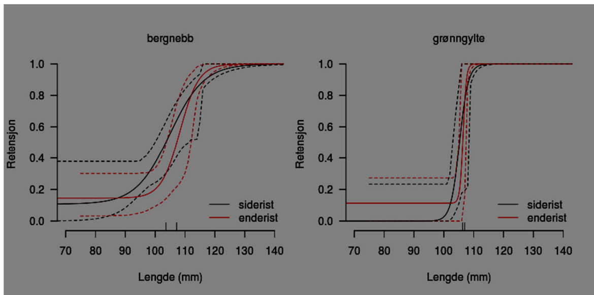
Figur 5. Siderist vs enderist. Estimerte seleksjonskurver for bergnebb (venstre) og grønnngylte (høyre). Heltrukne linjer angir seleksjonskurven og de stiplede angir tilhørende 95% konfidensregion.
