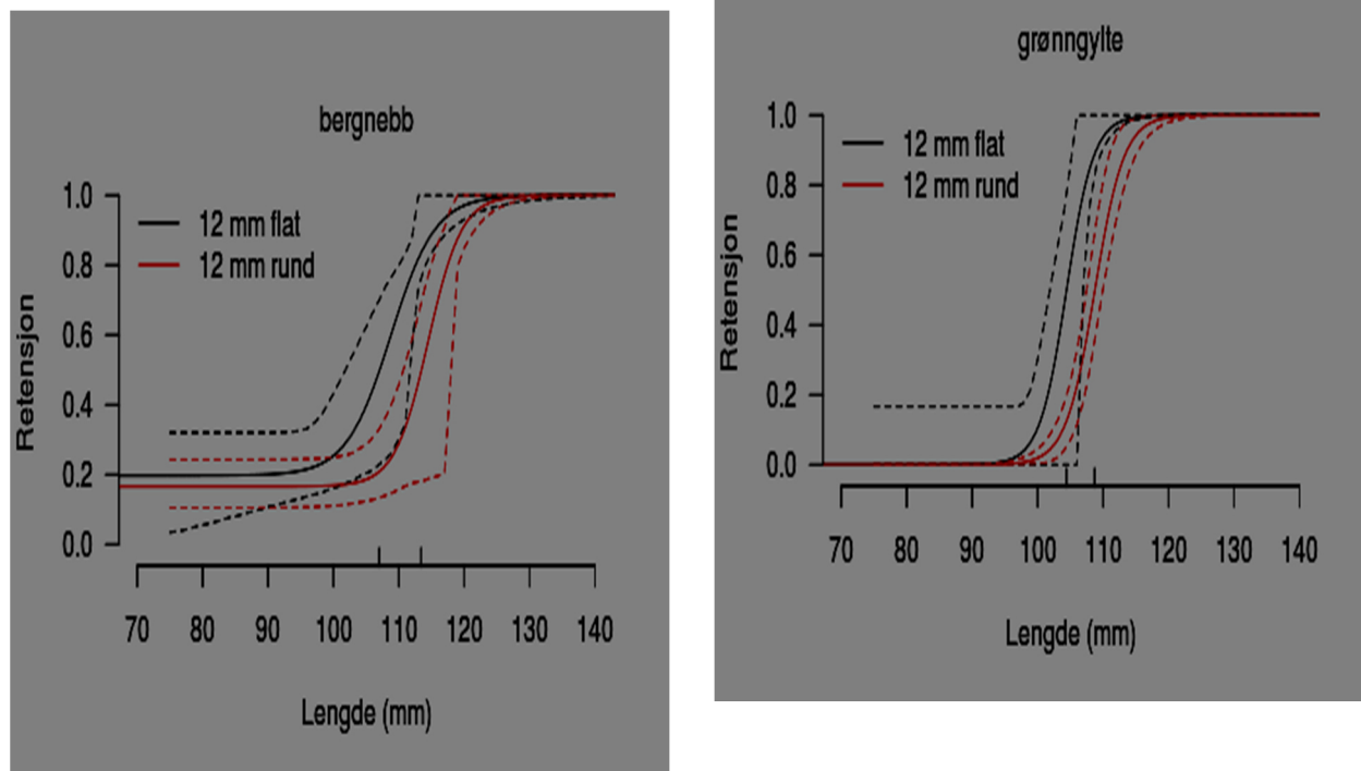
Figur 7. Flate vs runde spiler i rist med 12 mm spaltebredde. Estimerte seleksjonskurver for bergnebb (venstre) og grønngylte (høyre). Heltrukne linjer angir seleksjonskurven og de stiplede angir tilhørende 95% konfidensregion.
