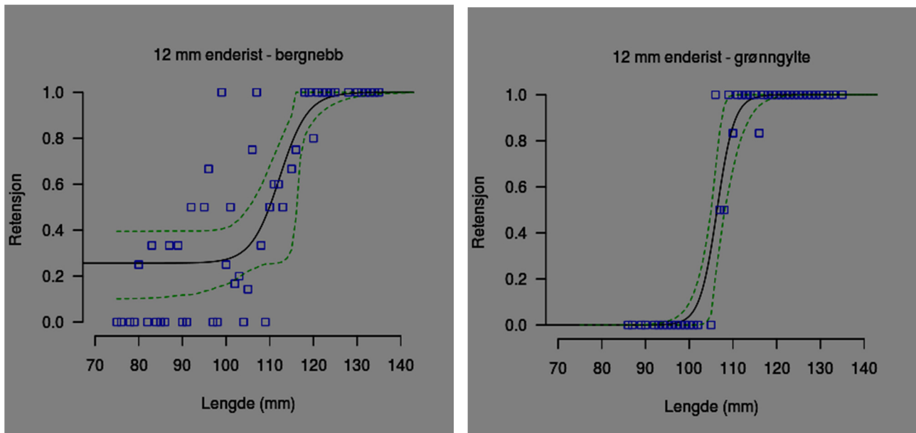
Fig. 4. Eksempel på forskjell i kontaktsannsynlighet med sorteringsrist med 12 mm spaltebredde for bergnebb (venstre) og grønngylte (høyre).
