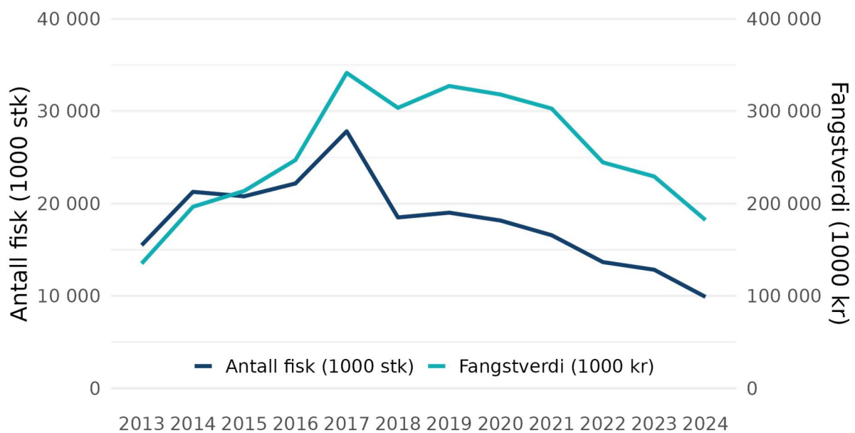
Figur 2.1: Fangst (antall, 1000 stk.) og verdi (1000 kr) av leppefisk i perioden 2013-2024
