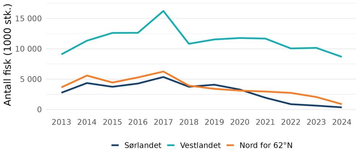
Figur 2.2: Fangst (antall, 1000 stk.) fordelt på de tre geografiske områdene i perioden 2013-2024
