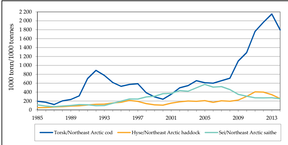
Figur 2B Gytebestand for nordaustarktisk torsk, nordaustarktisk hyse og nordaustarktisk sei nord for 62° N. 1985-2014.
