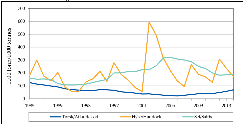
Figur 2C Gytebestand for torsk, hyse og sei i Nordsjøen og Skagerrak. 1985-2014.
