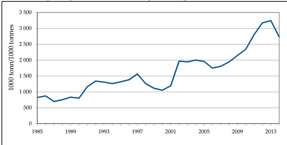
Figur 2A Gytebestand. Alle sentrale botnfiskartar 1) . 1985-2014.
